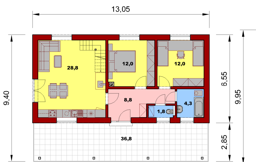
PŮDORYS PŘÍZEMÍ:
