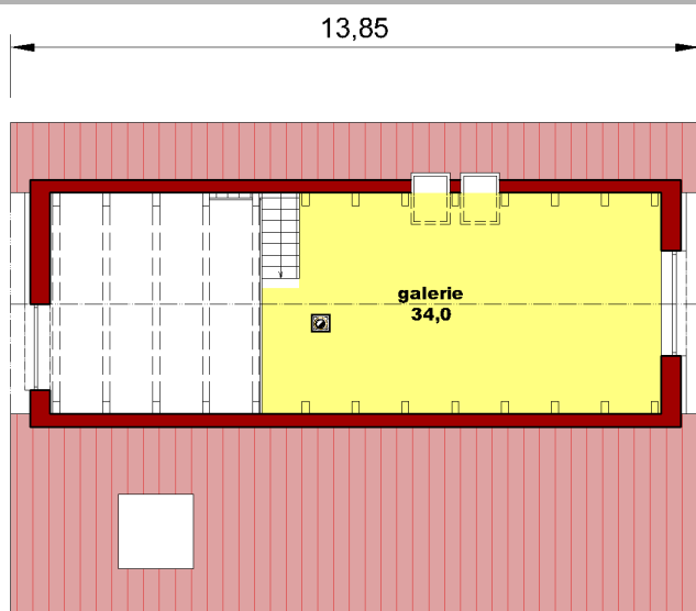
PŮDORYS GALERIE:
